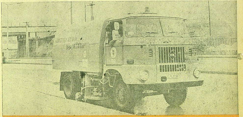
Az IFA gyár közelmúltban kifejlesztett nagy teljesítményű önteljesedő seprőgépe melián keltetettel a hazai szakembereink érdeklődését. Az óránkint 35 ezer négyzetméternyi seprési teljesítményre képes gép 4,5 köbméteres gyűjtőtartállyal, a 2300 milliméteres, illetve 2900 milliméteres seprési szélességgel igen jól helyettesíti a hasonló népek versenyében.
